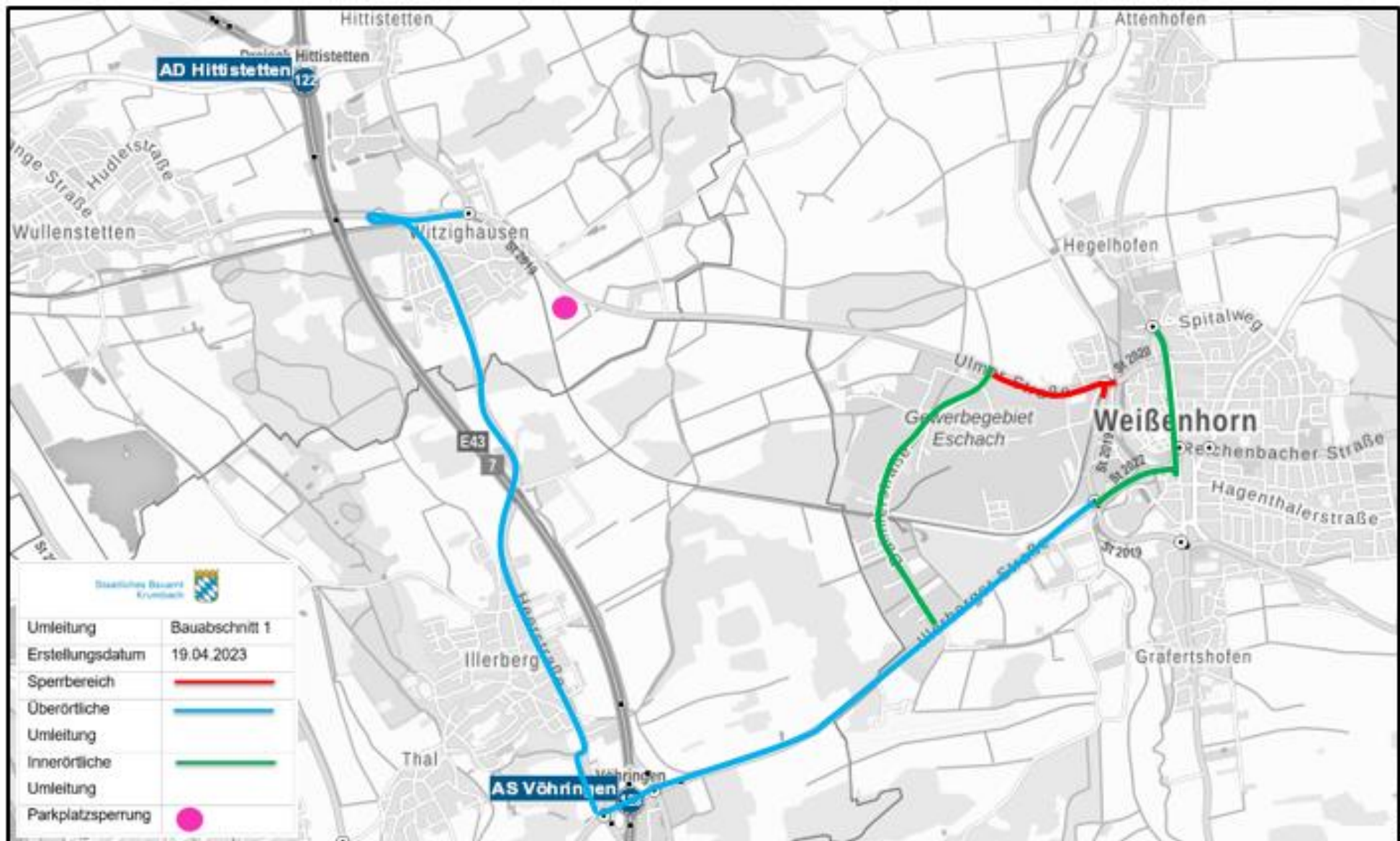
Abbildung 3 Umleitungsplan Bauabschnitt 1
